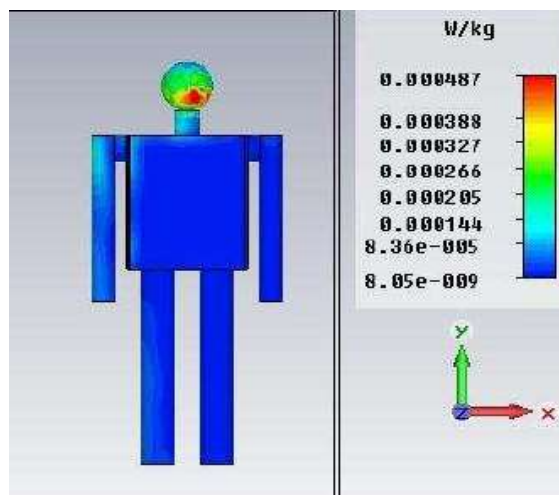
شکل ۳- میزان جذب انرژی در بدن در میدان دور
