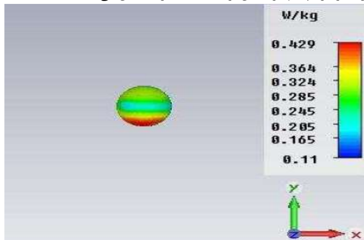
شکل ۲- میزان جذب انرژی در کره چشم در میدان نزدیک
