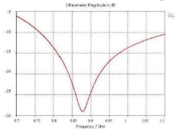
نمودار ۱- پارامتر S_{11}
