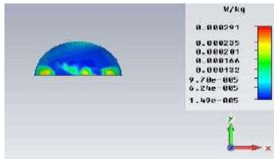
شکل ۶- میزان جذب انرژی در مغز در میدان دور
