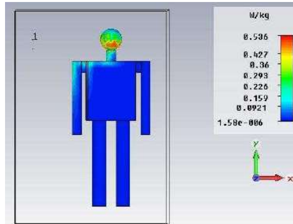
شکل ۲- میزان جذب در بدن انسان در میدان نزدیک
