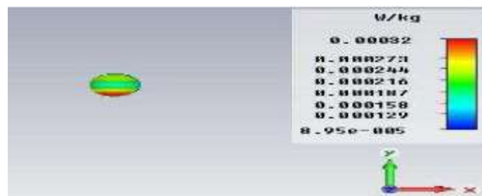
شکل ۷- میزان جذب انرژی در چشم در میدان دور
