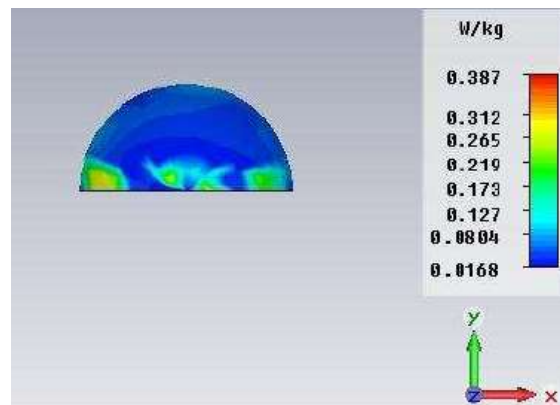
شکل ۳- میزان جذب انرژی در مغز در میدان نزدیک
