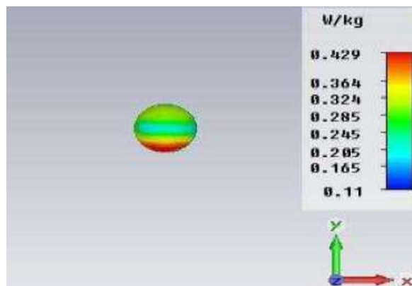
شکل ۴- میزان جذب انرژی در کره چشم در میدان نزدیک
